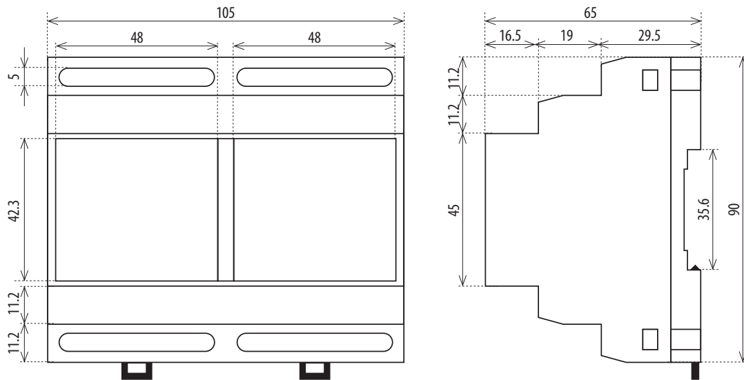
6-MODUL
