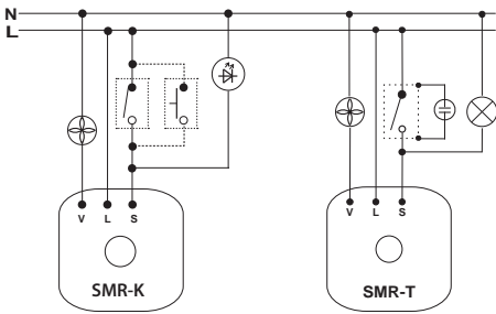
Typické zapojení SMR-K, - časovač pro ventilátor
